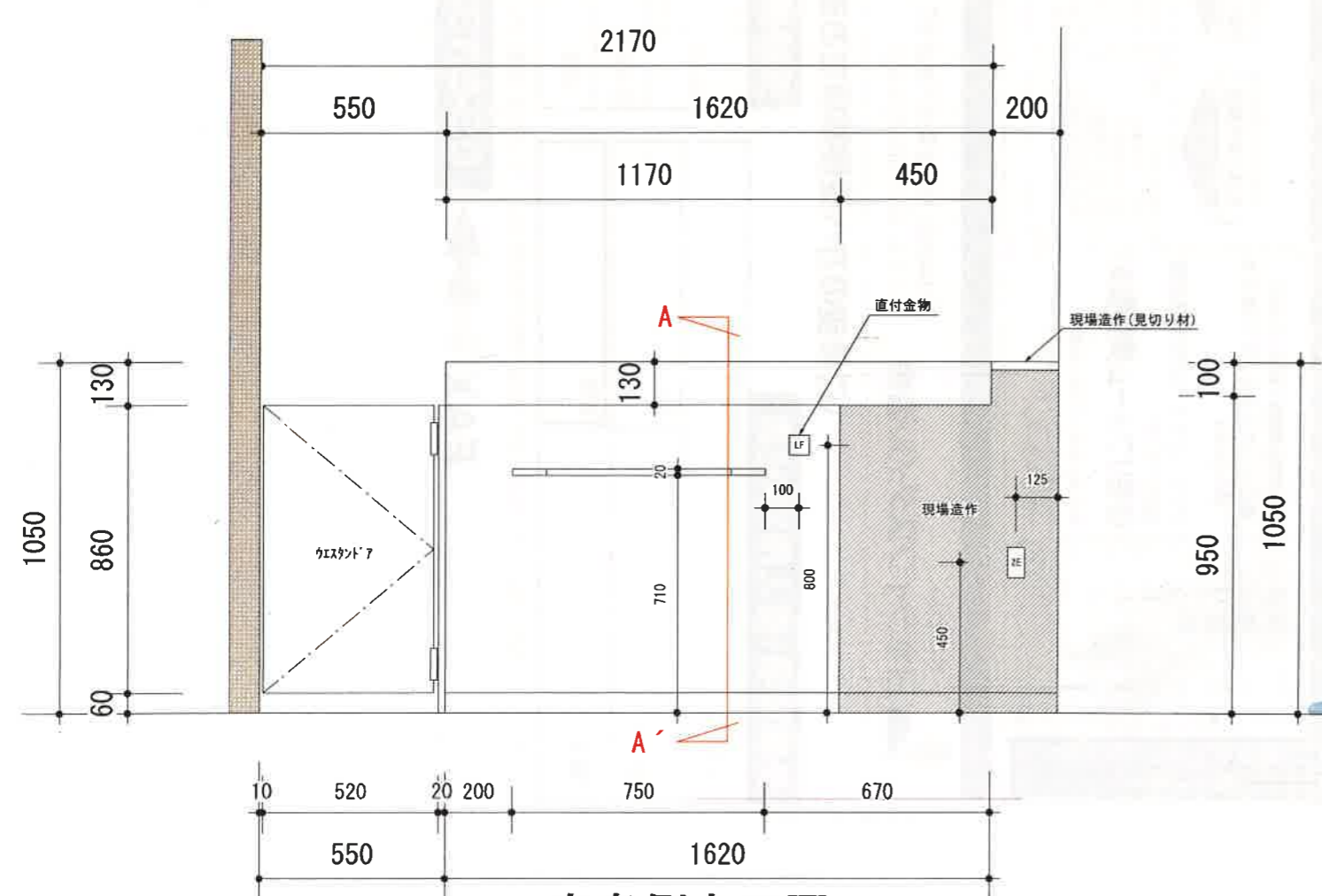
患者側立面図
