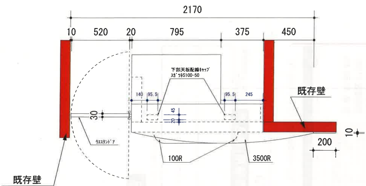
上面図
