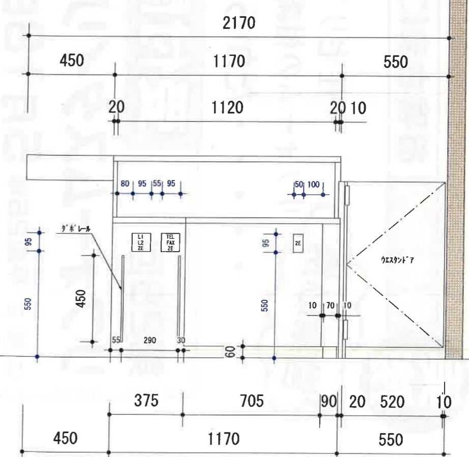
従業員側立面図
